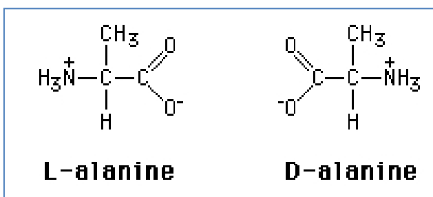
Fig. 4.1 : Enantiomer isomers of amino acids
