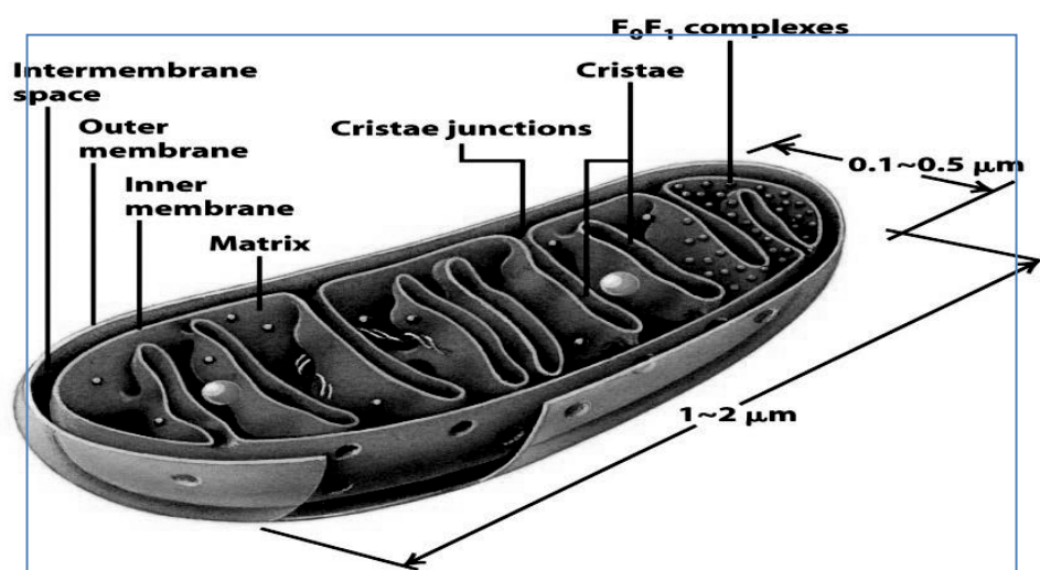
Fig. 2.2 : Structure of mitochondria
