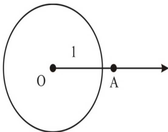
Fig.: circle r = 1
