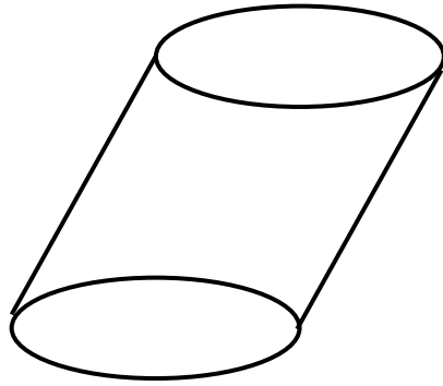
Fig. 5.5 (Oblique Circular Cylinder)
