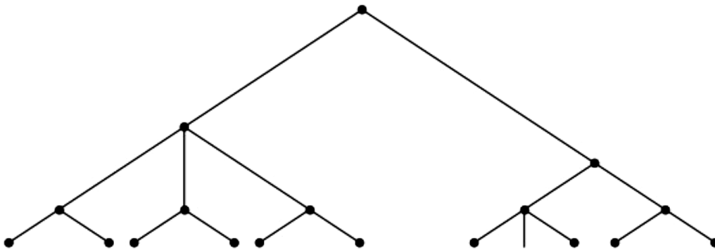
Fig. 10 B-tree
