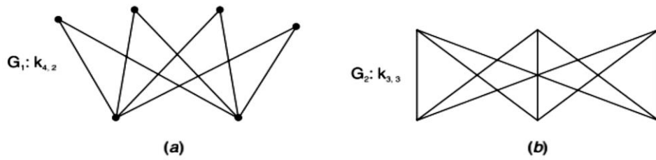
Fig.18 complete bipartite
