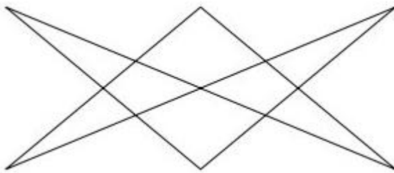
Fig.17 Bipartite graph
