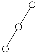
Left Skew
