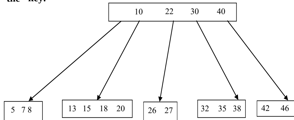
Step 2
