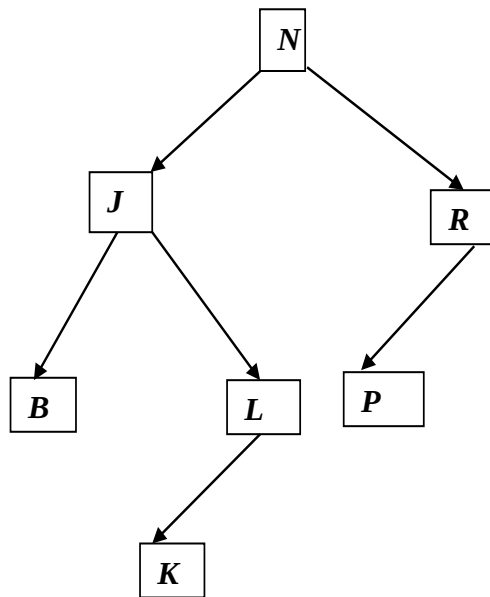
Step 6
